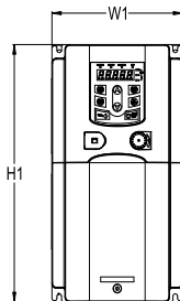
그림 B-3 0R7G-015G/018P 벽걸이형 설치 설명도 (단위: mm)
