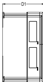
그림 B-3 0R7G-015G/018P 벽걸이형 설치 설명도 (단위: mm)
