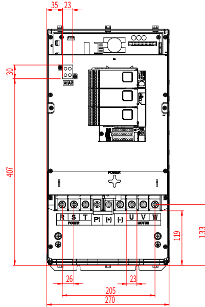
그림 4-21 380V 037G/045P-055G/075P 메인 회로 단자
