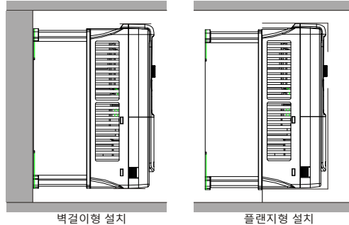
그림 4-2 설치 방법
