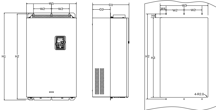
그림 B-11 132G/160P~200G/220P 플랜지형 설치 설명도 (단위: mm)
