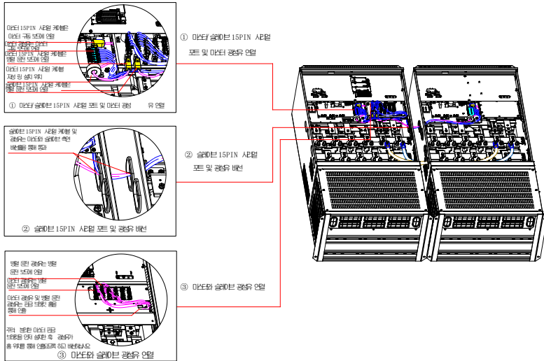
그림 4-10 마스터와 슬레이브 연결도 1 (560kW~630kW)
