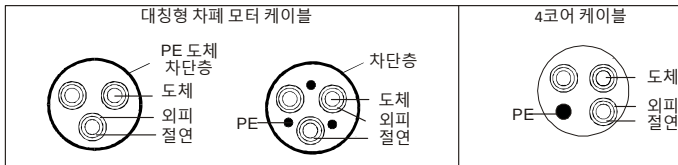
그림 C-1 대칭형 차폐 모터 케이블
