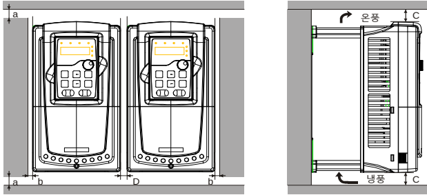
그림 4-3 병렬 설치
