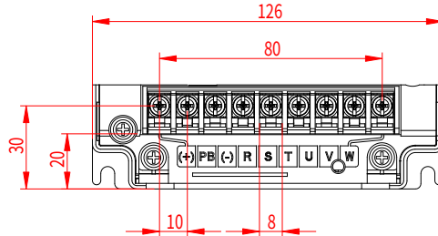
그림 4-16 380V 0R7G-2R2G 메인 회로 단자
