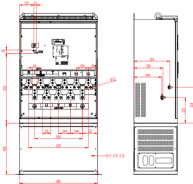
그림 4-23 380V 132G/160P-200G/220P 메인 회로 단자
