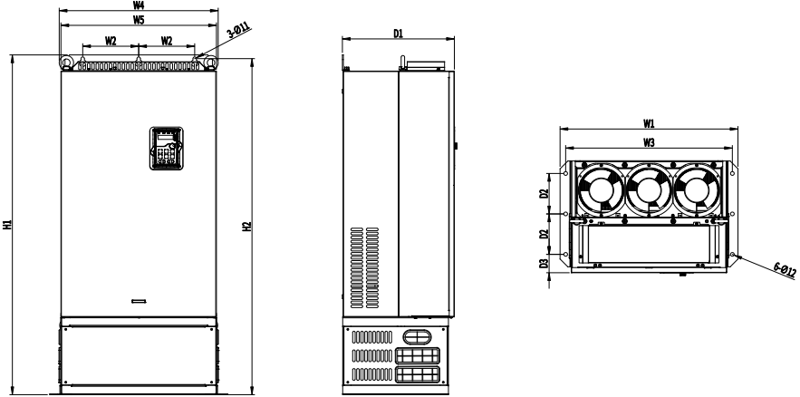
그림 B-12 132G/160P-200G/220P 바닥형 설치 설명도 (단위: mm, 베이스 포함)
