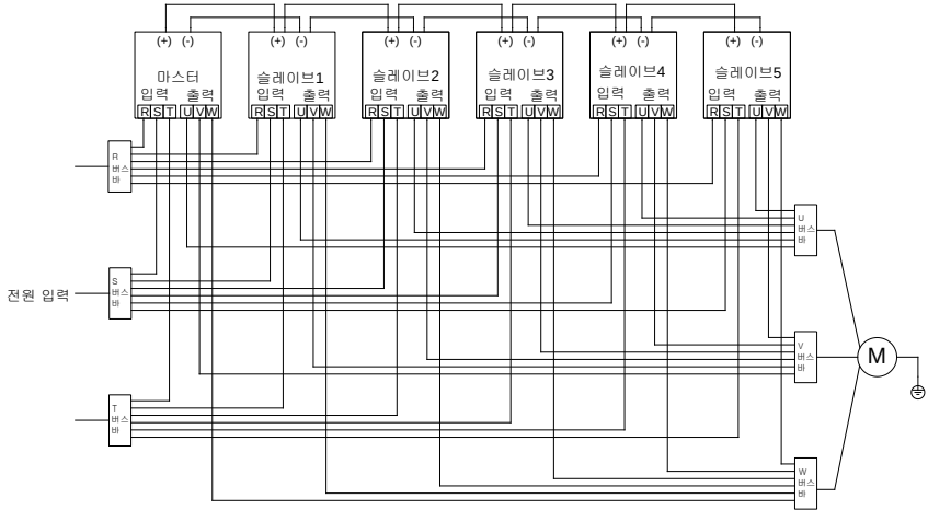
그림 4-9 병렬 주 회로 배선
