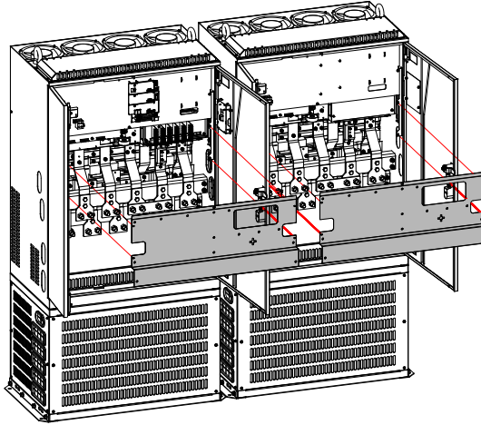
그림 4-12 판금 브래킷 분리도
