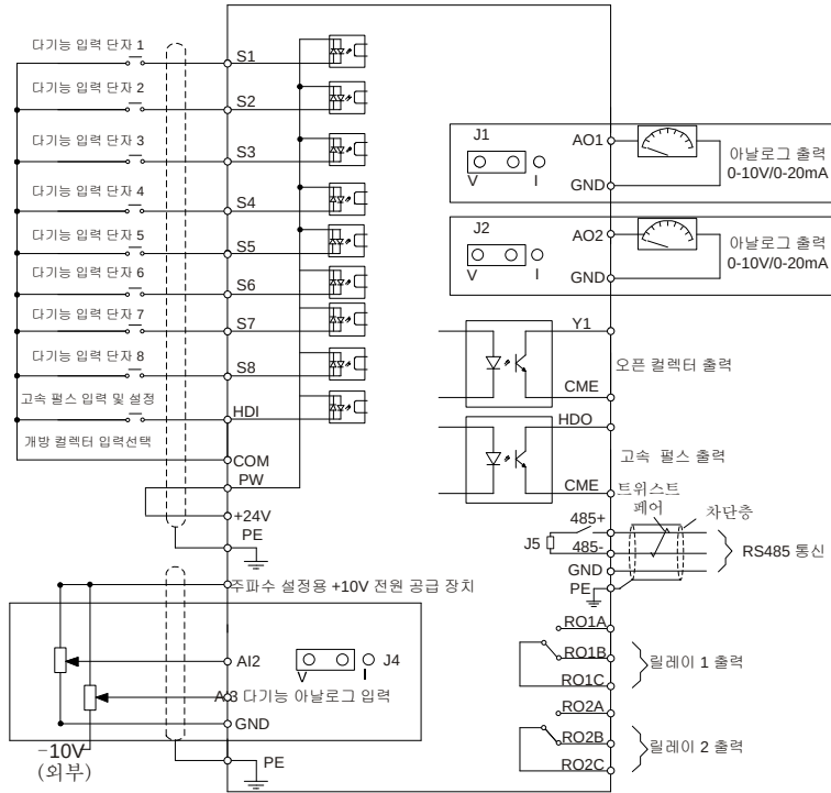
그림 4-29 제어 회로 배선도
