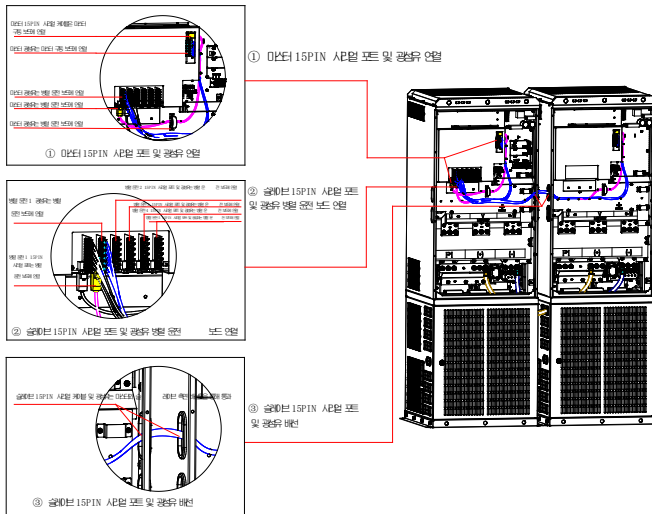
그림 4-13 마스터와 슬레이브 연결도 1 (710kW~3000kW)
