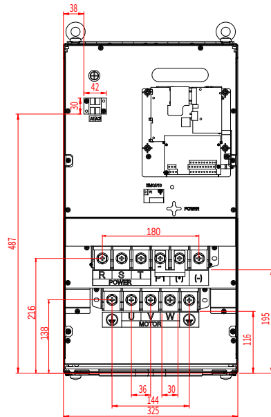
그림 4-21 380V 037G/045P-055G/075P 메인 회로 단자
