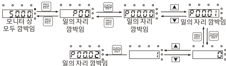
그림 5-5 매개 변수 설명 도면
