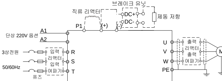
그림 4-8 380V 037G/045P 급 이상의 메인 회로 배선도
