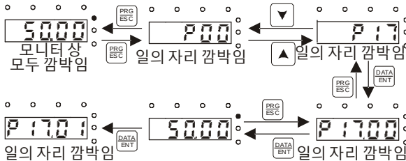
그림 5-7 매개 변수 설명도
