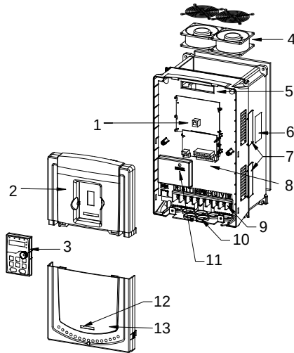
그림 3-6 제품구성도
