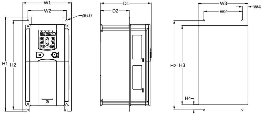
그림 B-8 0R7G-015G/018P 플랜지형 설치 설명도 (단위: mm)
