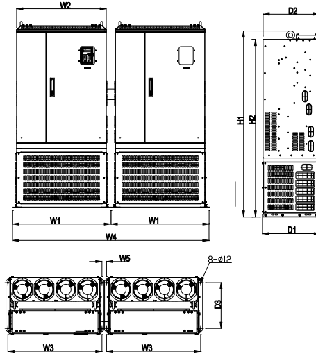
그림 B-15 380V 560~630kW 병렬 설치
