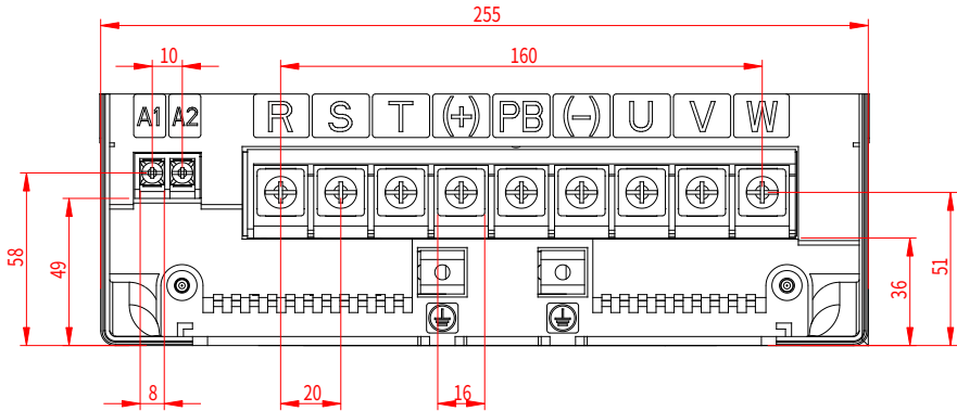
그림 4-20 380V 022G/030P-030G/037P 메인 회로 단자
