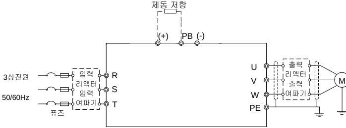
그림 4-6 380V 5R5G/7R5P 급 이하의 메인 회로 배선도
