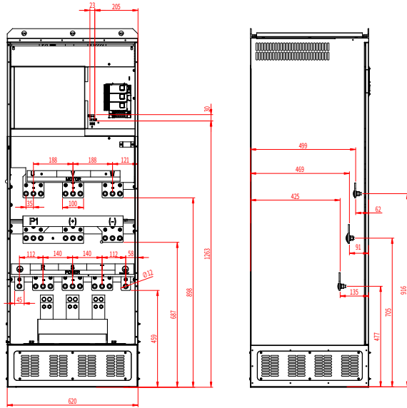
그림 4-25 380V 355G/400P-500G 메인 회로 단자
