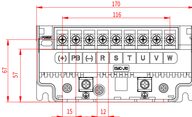
그림 4-18 380V 7R5G/011P-015G/018P 메인 회로 단자
