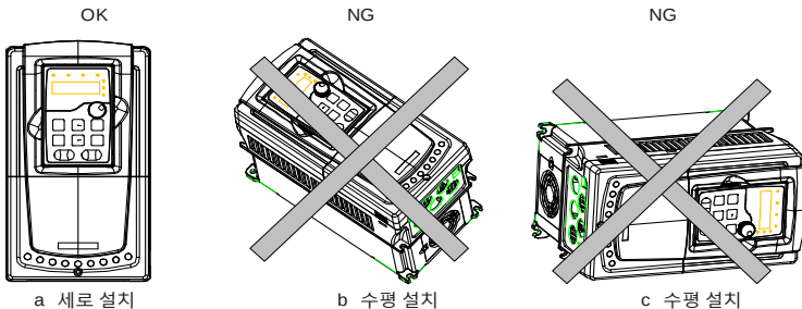
그림 4-1 인버터 설치 방향
