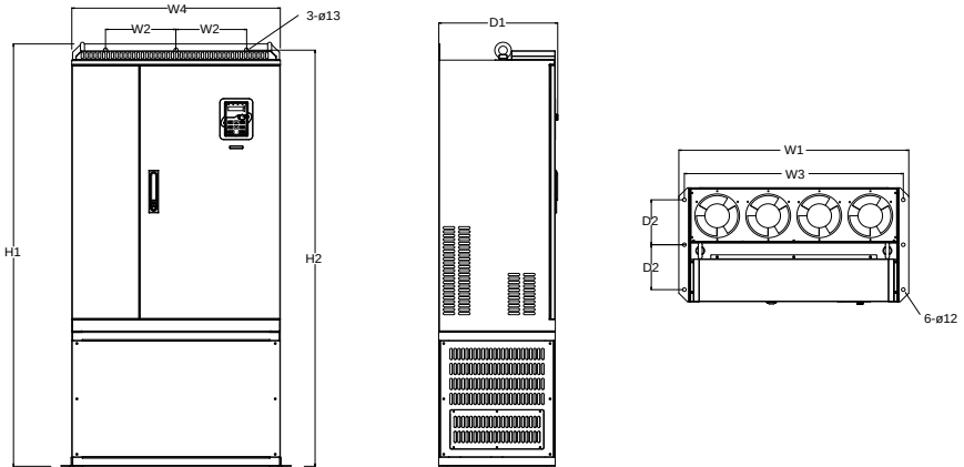
그림 B-13 220G/250P-315G/355P 바닥형 설치 설명도 (단위: mm, 베이스 포함)
