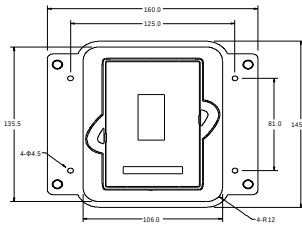
키패드 변환 브래킷
