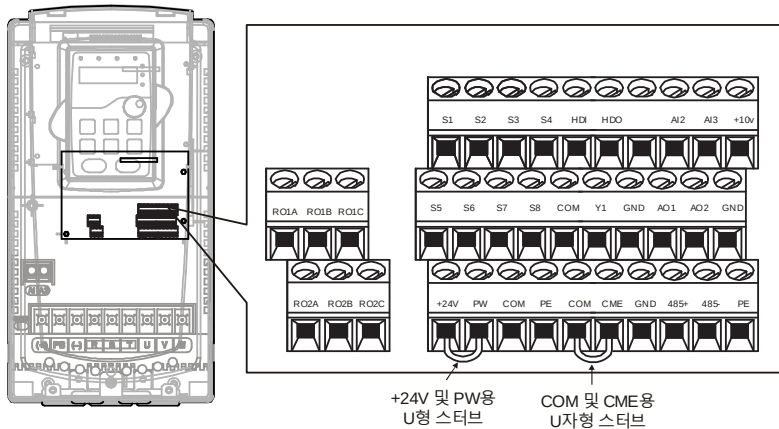
그림 4-34 380V 018G/022P 급 이상의 U 자형 단락 위치 설명도
