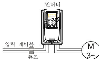
그림 4-37 퓨즈 배치도
