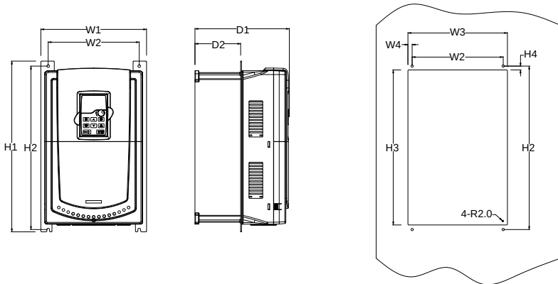
그림 B-9 018G/022P-030G/037P 플랜지형 설치 설명도 (단위: mm)
