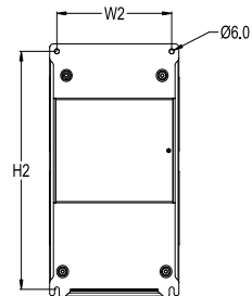
그림 B-3 0R7G-015G/018P 벽걸이형 설치 설명도 (단위: mm)
