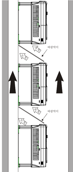
그림 4-4 수직 설치
