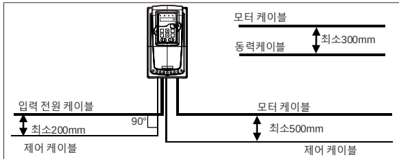
그림 C-4 배선거리
