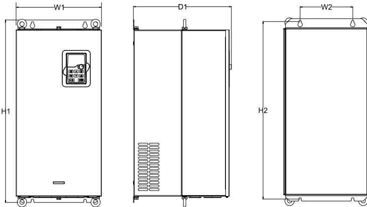
그림 B-5 037G/045P-110G/132P 벽걸이형 설치 설명도 (단위: mm)
