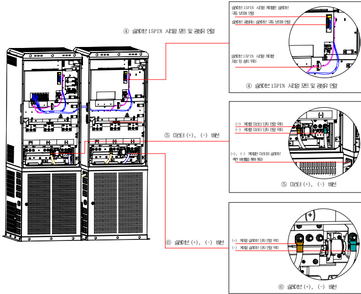
그림 4-14 마스터와 슬레이브 연결도 2 (710kW~3000kW)
