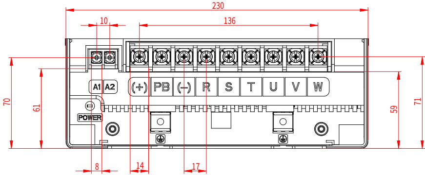
그림 4-19 380V 018G/022P 메인 회로 단자
