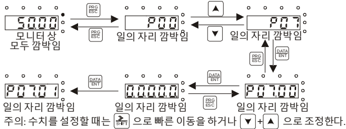
그림 5-6 비밀번호 설정 설명도
