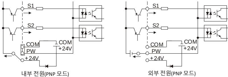
그림 4-36 PNP 모드 도면
