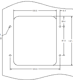
고객 설치 치수
