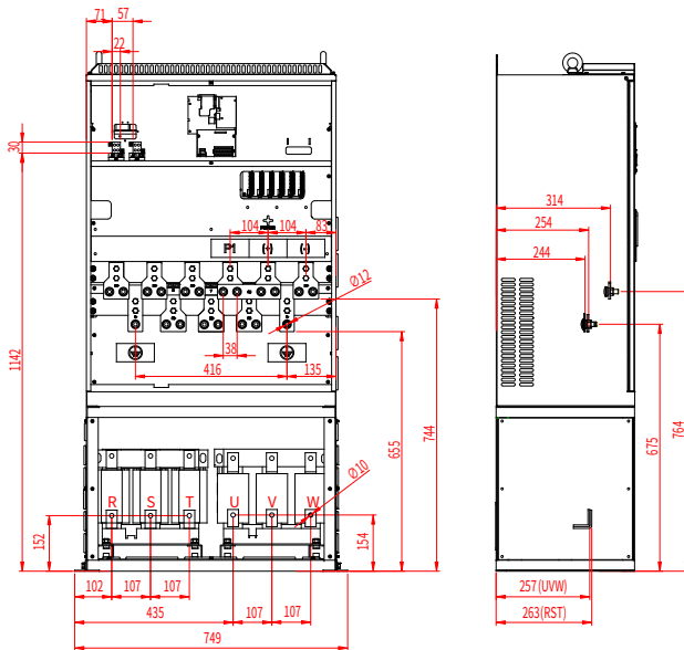
그림 4-26 380V 560G-630G 메인 회로 단자
