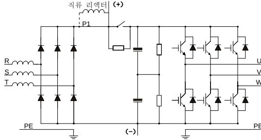
그림 3-3 380V 355G/400P 급 이상 메인 회로 약도
