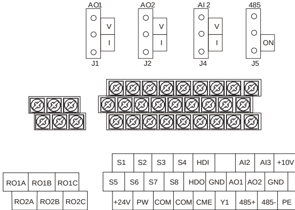
그림 4-31 380V 015G/018P 급 이하의 제어 단자 설명도
