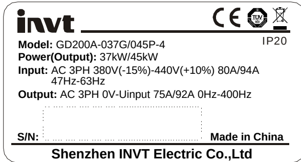
그림 3-4 제품 명판
