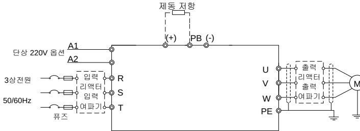
그림 4-7 380V 7R5G/011P-030G/037P 주회로 배선도
