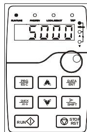
작동 파라미터 상태 표시
