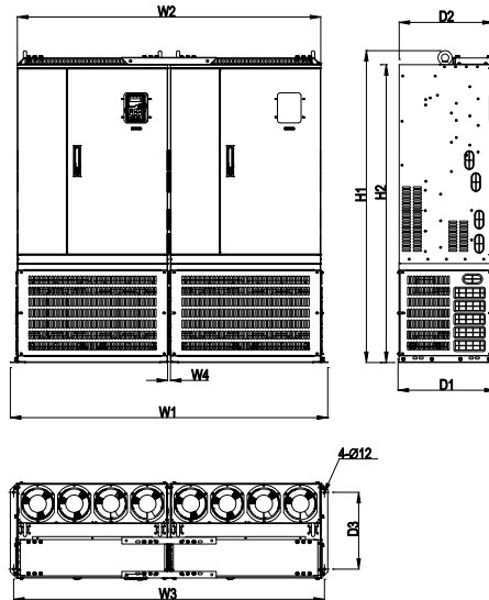
그림 B-17 380V 560~630kW 병렬 설치
