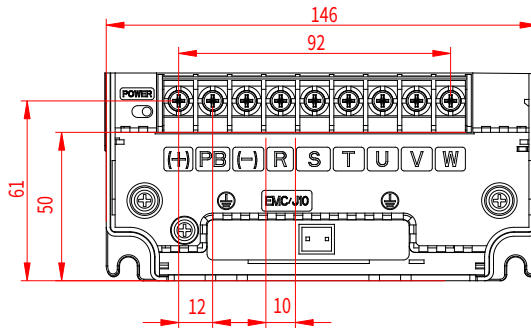
그림 4-17 380V 004G/5R5P-5R5G/7R5P 메인 회로 단자
