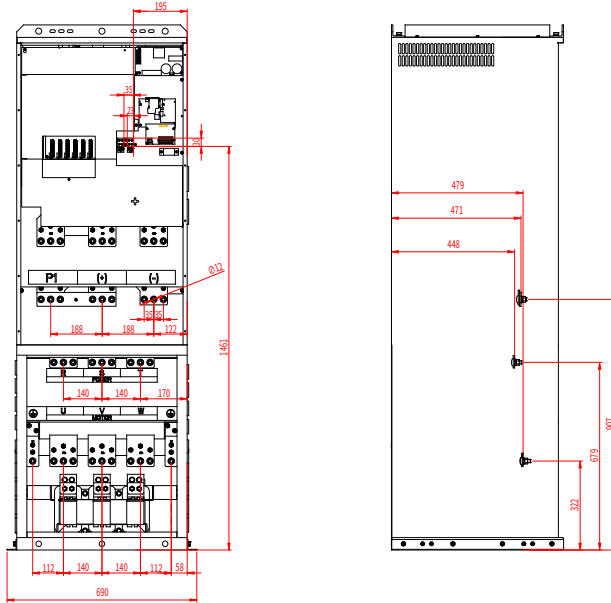
그림 4-27 380V 710G-3000G 메인 회로 단자
