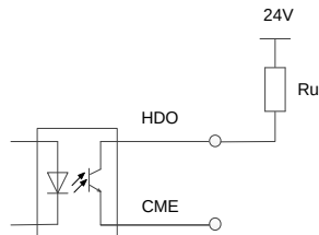
그림 4-30 HDO 접선 설명도
