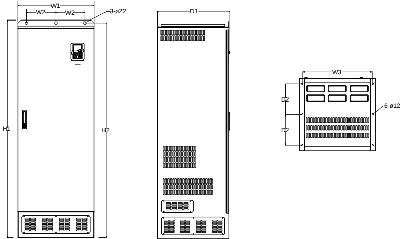
그림 B-14 355G/400P-500G 바닥형 설치 설명도 (단위: mm, 베이스 포함)
