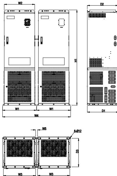
그림 B-16 380V 710~3000kW 병렬 설치
