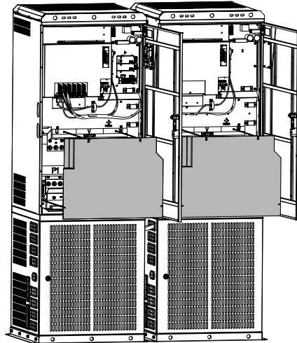
그림 4-15 투명 단자 커버 분리도
