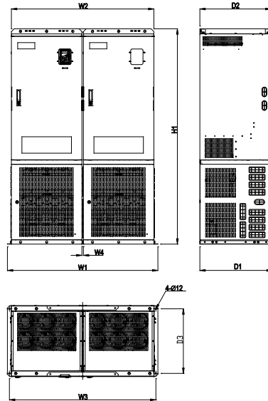
그림 B-18 380V 710~3000kW 병렬 설치
