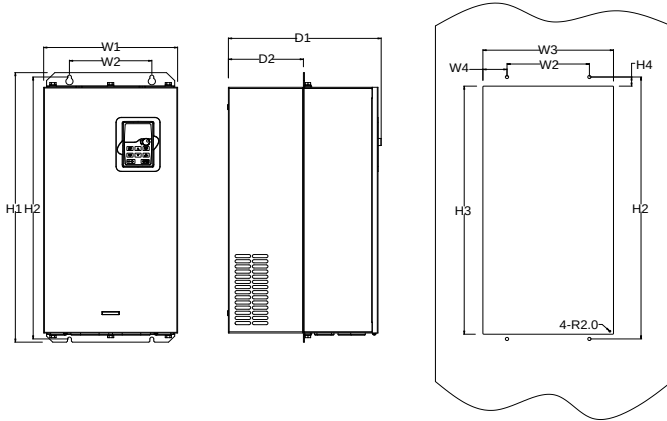
그림 B-10 037G/045P~110G/132P 플랜지형 설치 설명도 (단위: mm)
