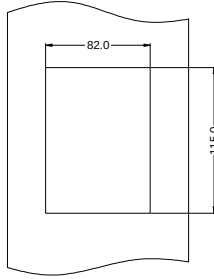
그림 B-1 키패드 거치대(옵션)
