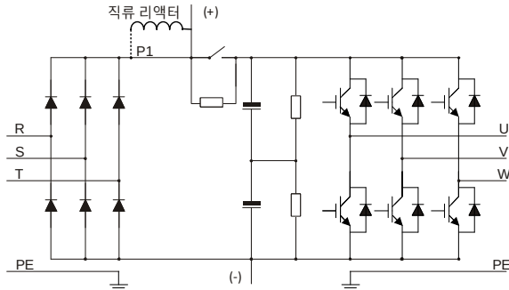
그림 3-2 380V 037G/045P~315G/355P 메인 회로 약도
