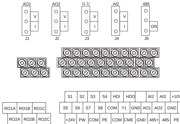
그림 4-32 380V 018G/022P 급 이상의 제어 단자 설명도
