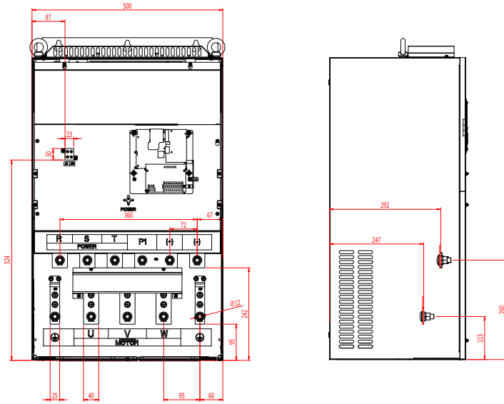
그림 4-23 380V 132G/160P-200G/220P 메인 회로 단자
