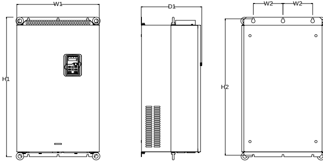
그림 B-6 132G/160P-200G/220P 벽걸이형 설치 설명도 (단위: mm)
