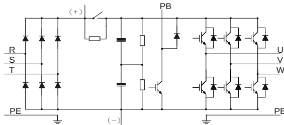
그림 3-1 380V 030G/037P 급 이하 메인 회로 약도
