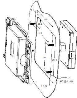
고객 설치 치수
