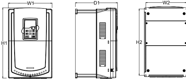
그림 B-4 018G/022P-030G/037P 벽걸이형 설치 설명도 (단위: mm)
