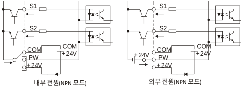
그림 4-35 NPN 모드 도면
