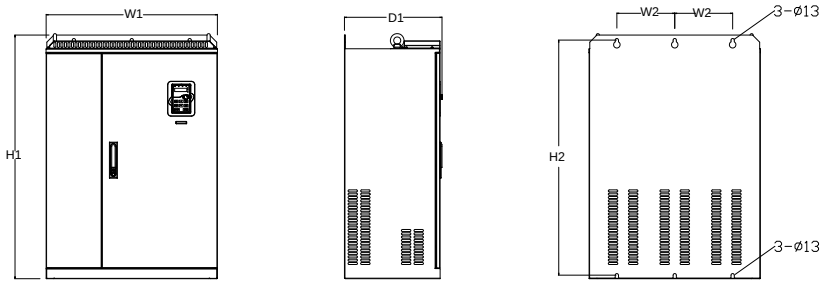
그림 B-7 220G/250P-315G/355P 벽걸이형 설치 설명도 (단위: mm)
