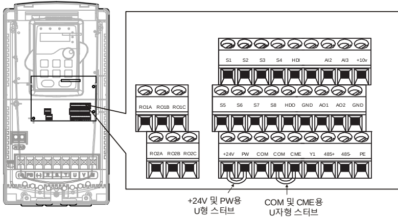
그림 4-33 380V 015G/018P 급 이하의 U 자형 단락 위치 설명도
