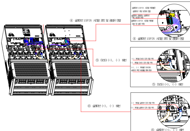
그림 4-11 마스터와 슬레이브 연결도 2 (560kW~630kW)
